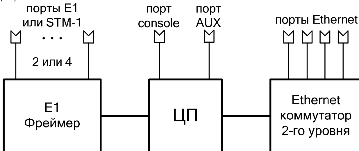
Рис. 9. Структурная схема шлюза ММ-104/ММ-116/ММ-164
