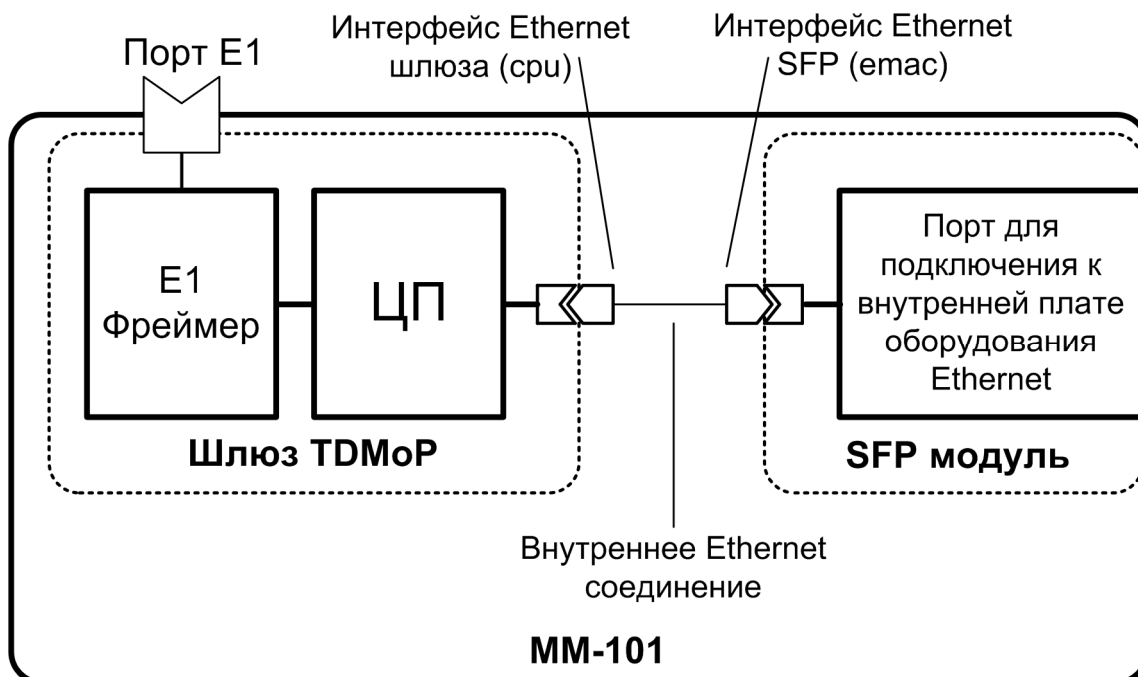
Рис. 11. Логическая схема шлюза MM-101
