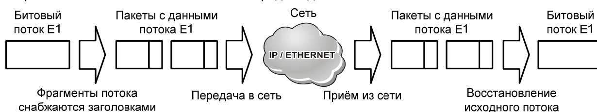
Рис. 7. Схема преобразования потока E1 при его передаче через пакетную сеть
