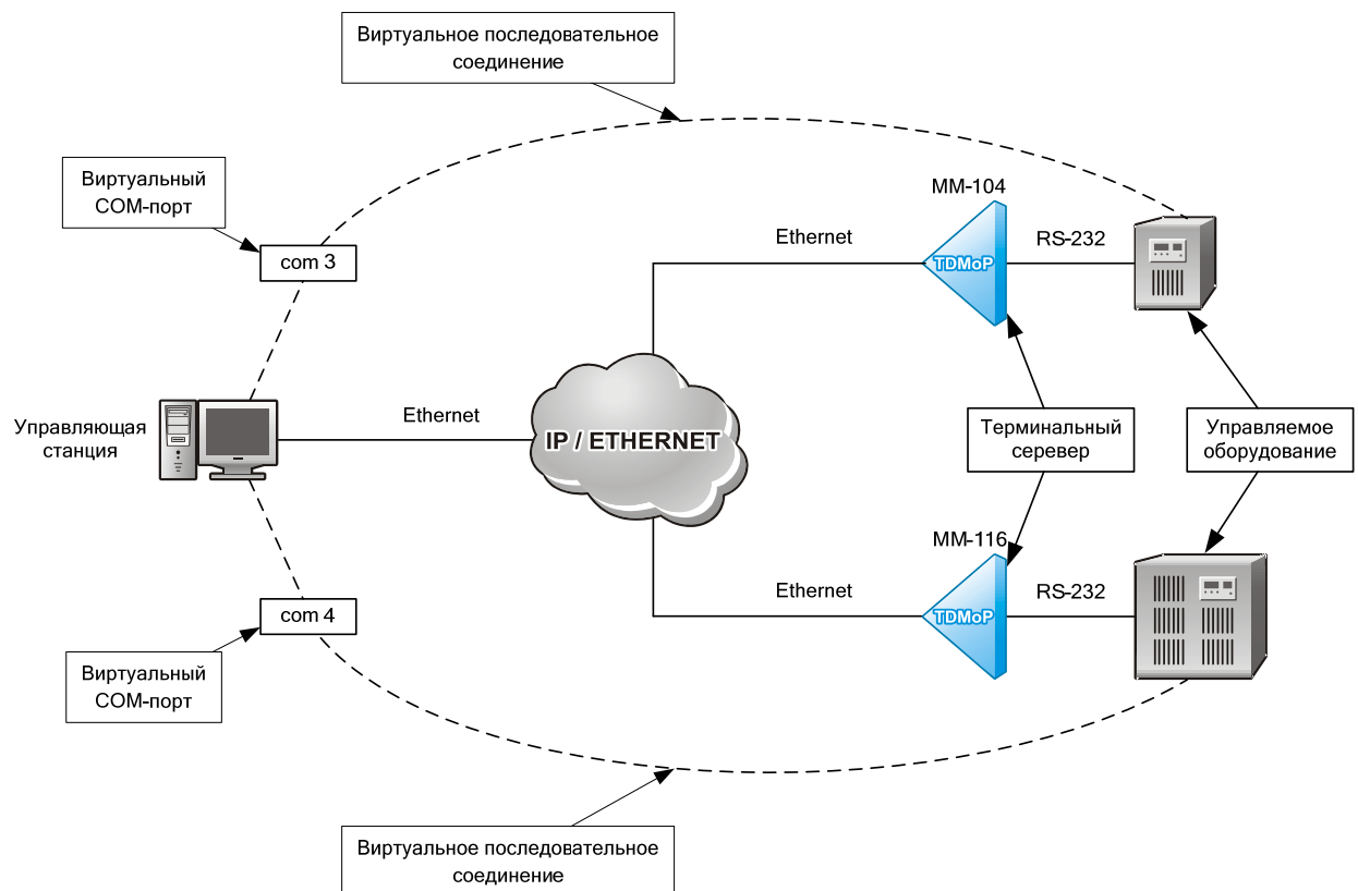
Рис. 12. Схема организации удаленного управления оборудованием по интерфейсу RS-232 через пакетную сеть при помощи встроенного терминального сервера
