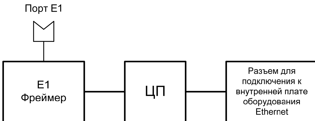
Рис. 10. Структурная схема шлюза ММ-101
