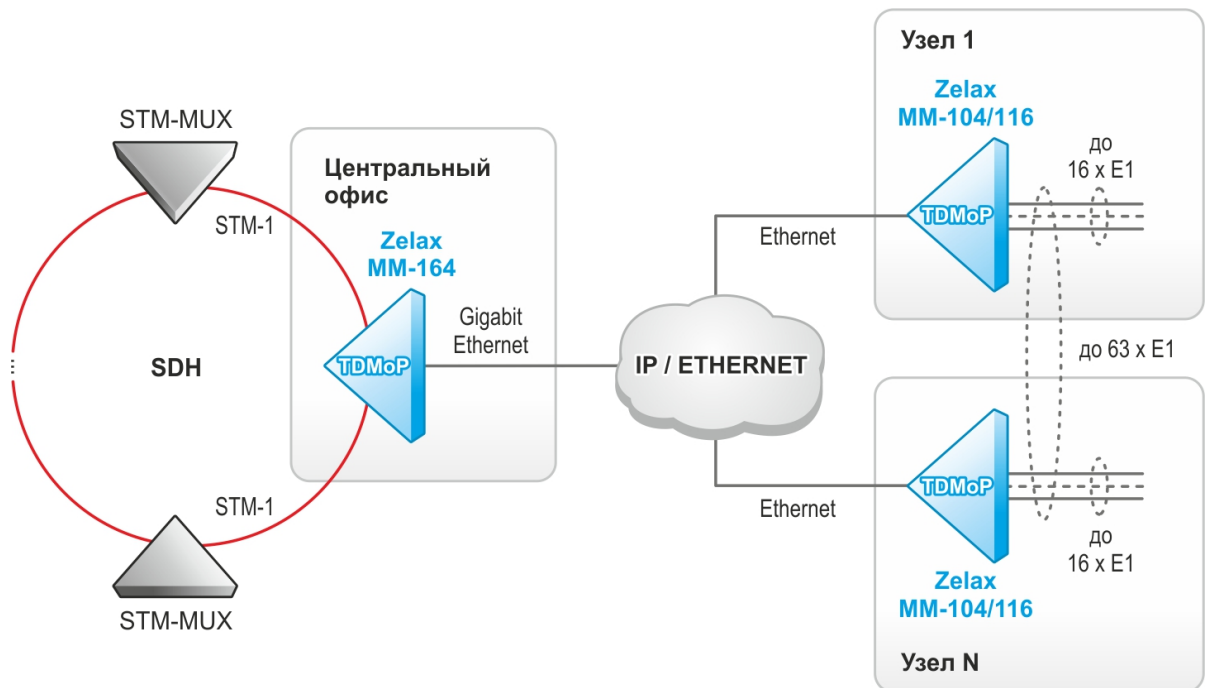
Рис. 5 Выделение/вставка до 63 потоков E1/G.703 из кольцевой сети SDH уровня STM-1 и передача их на оконечные узлы через сеть IP/Ethernet
