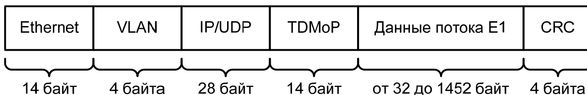
Рис. 8. Формат пакета с данными потока E1
