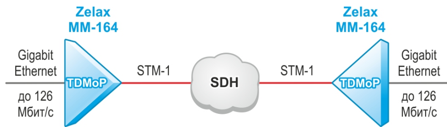
Рис. 6. Передача через сеть SDH данных Ethernet на скорости до 126 Мбит/с
